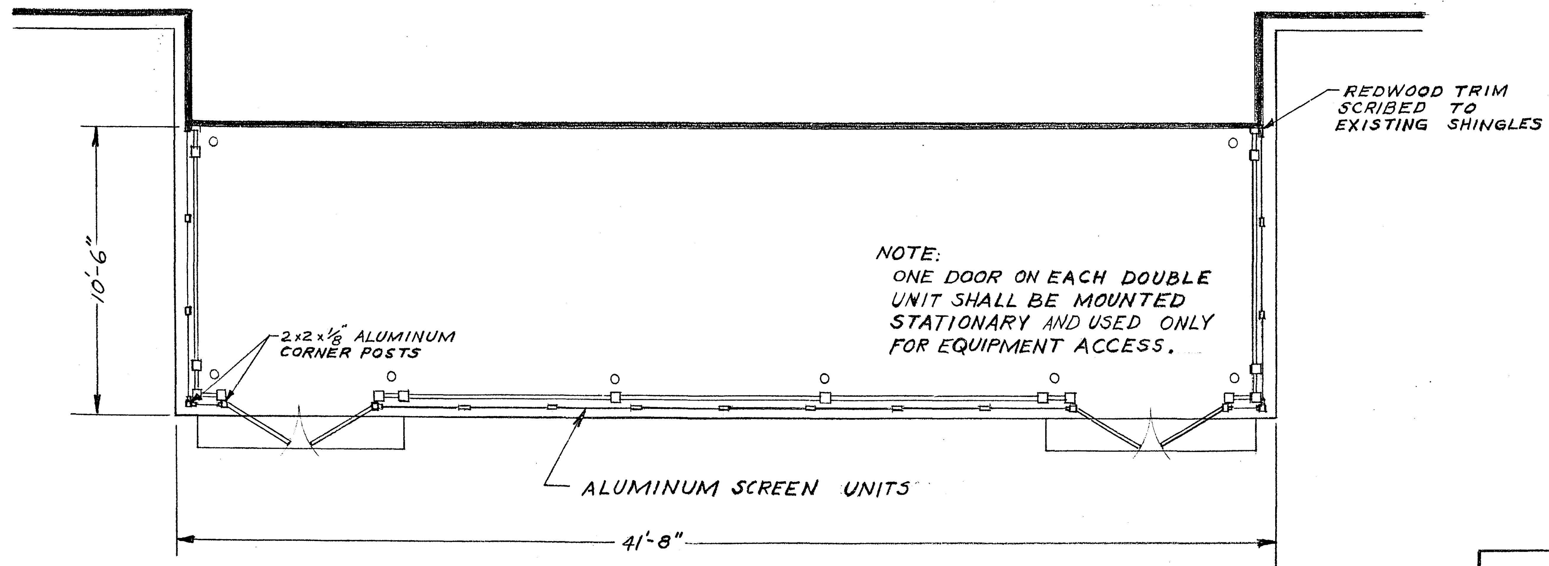
PLAN SCALE: 1/4" = 1'-0"
