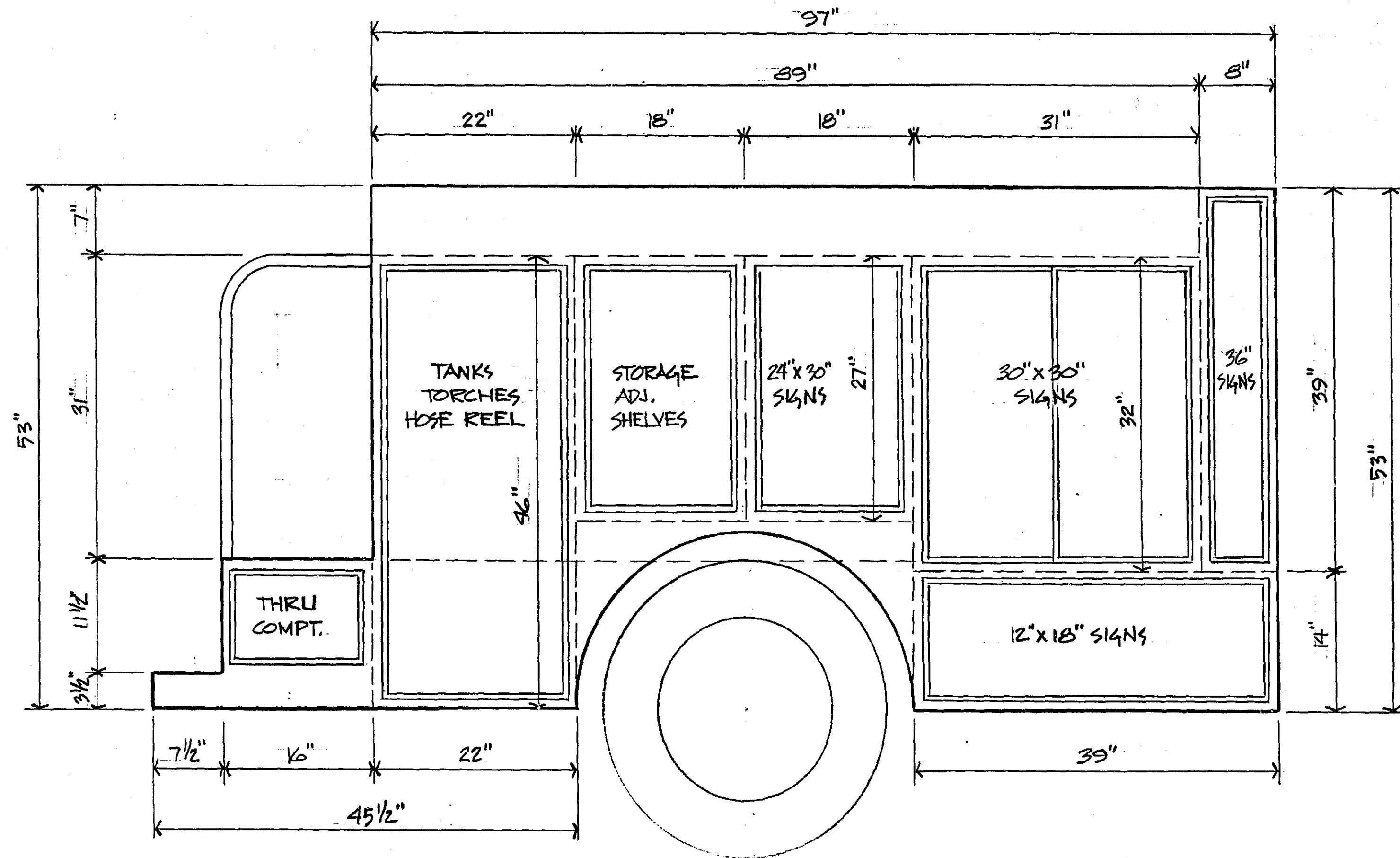
RIGHT SIDE VIEW SCALE: 1" = 1'-0"
