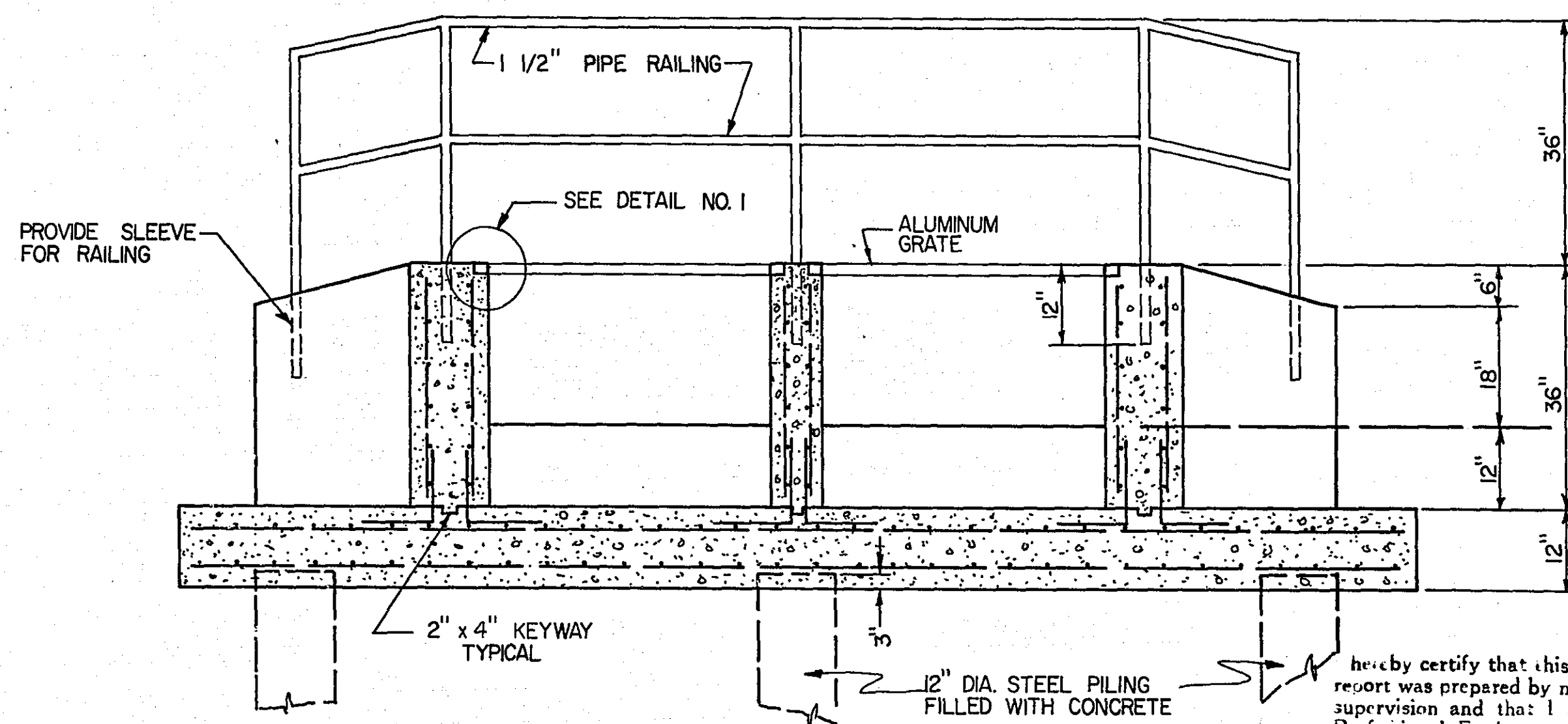
SECTION A-A
