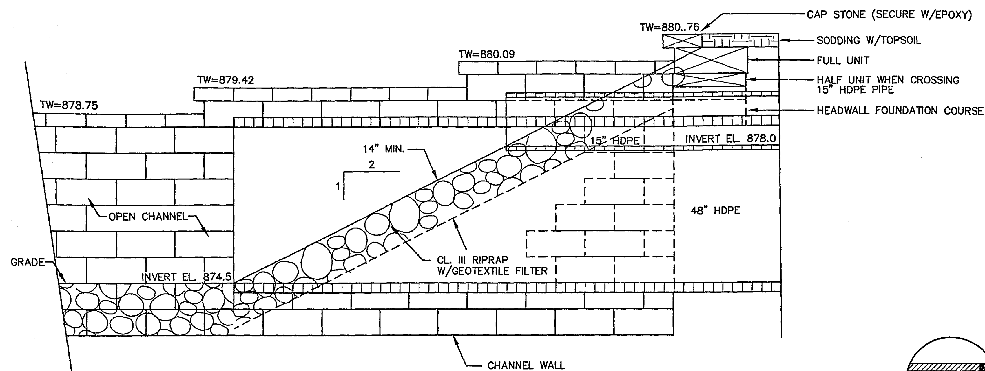
SECTION A-A N.T.S.
