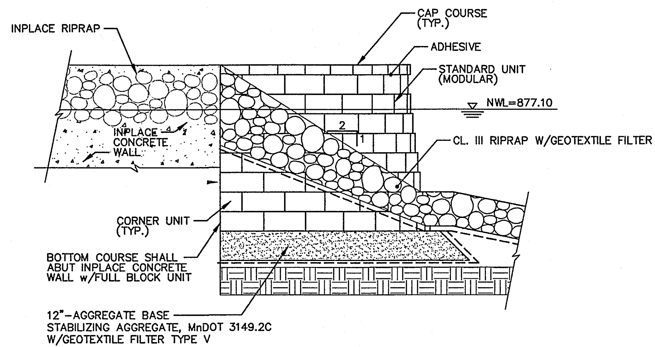
ELEVATION A-A N.T.S.
