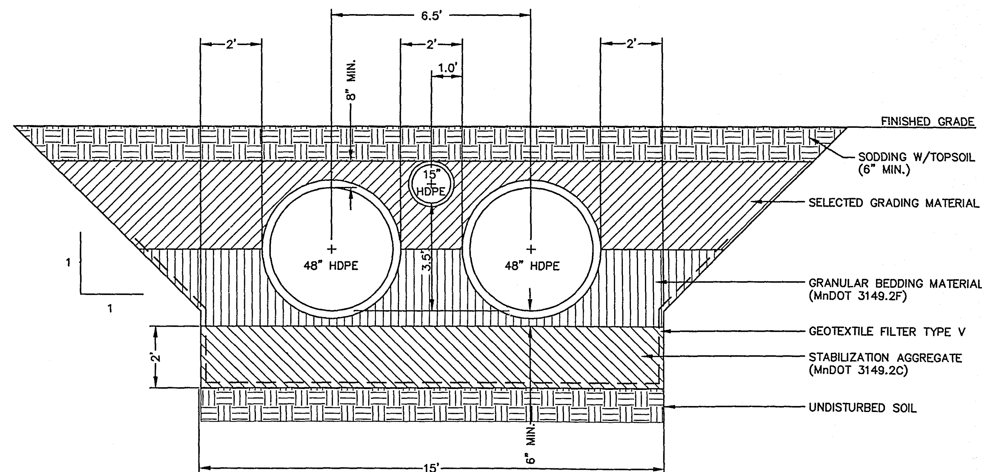
PIPE BEDDING DETAIL N.T.S.
