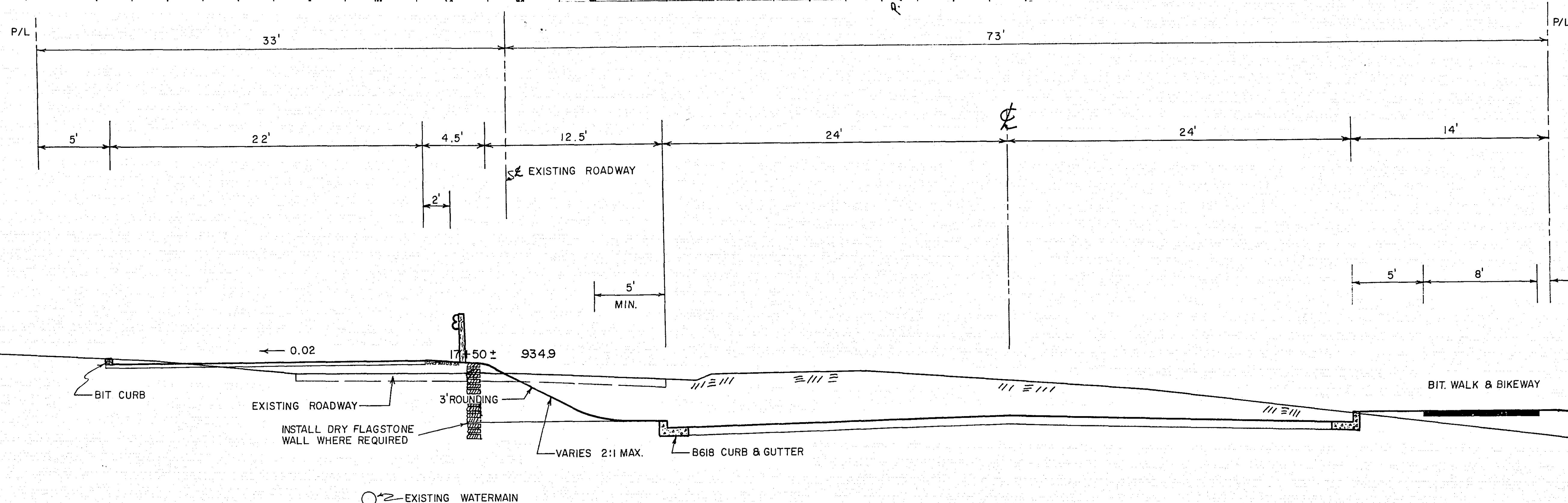
SECTION A-A
