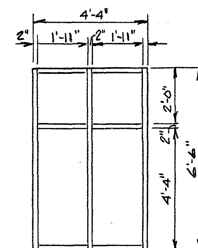
FRAME-6
