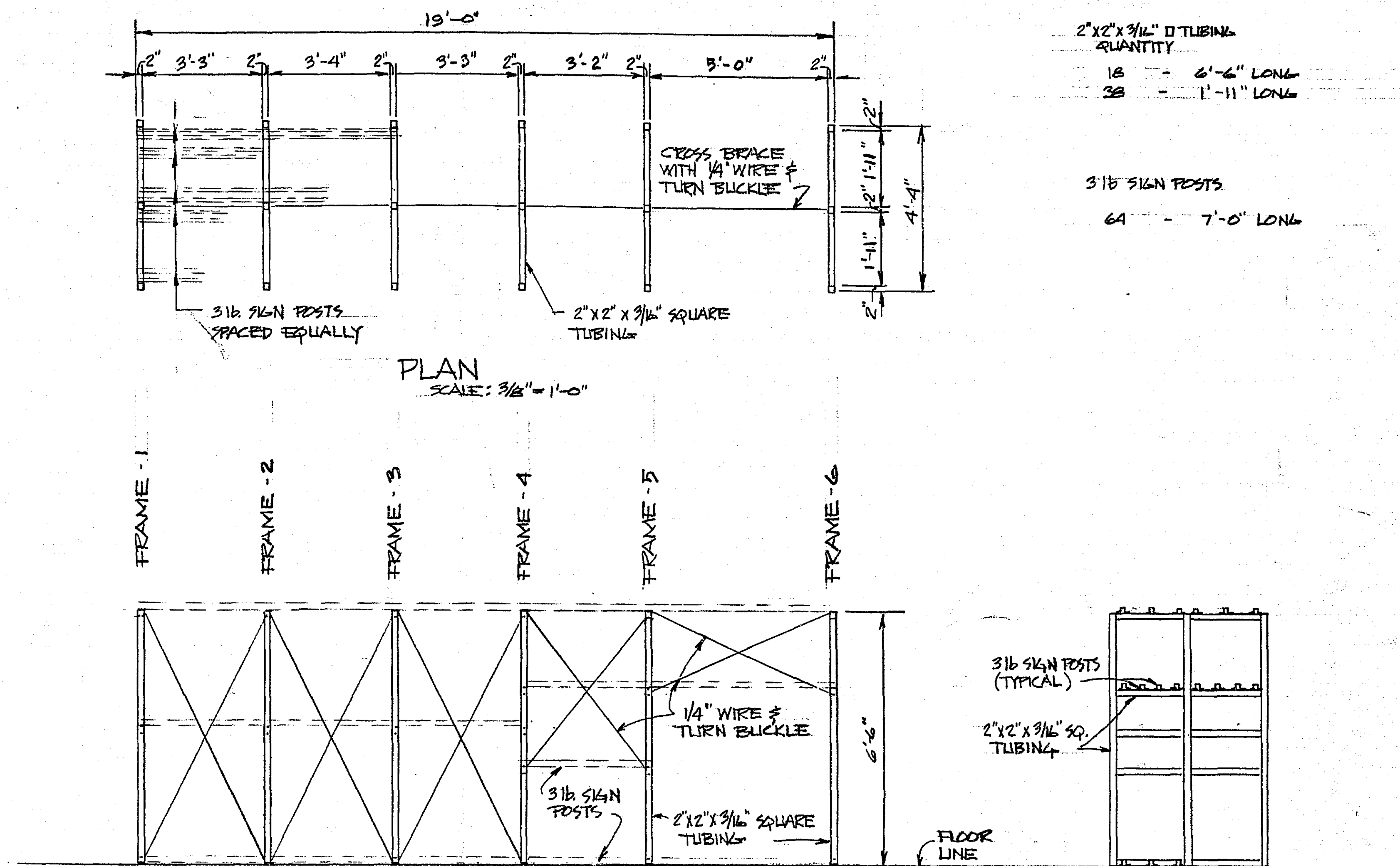
FRONT SCALE: 3/8" = 1'-0"
