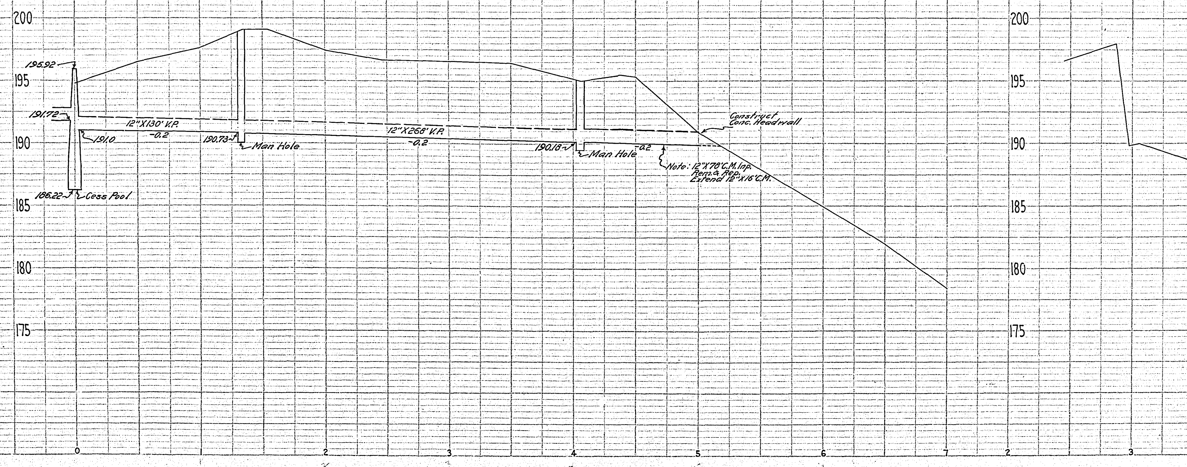
PLATE 1 - PLAN-PROFILE C. P. R. & H. C. STANDARD
